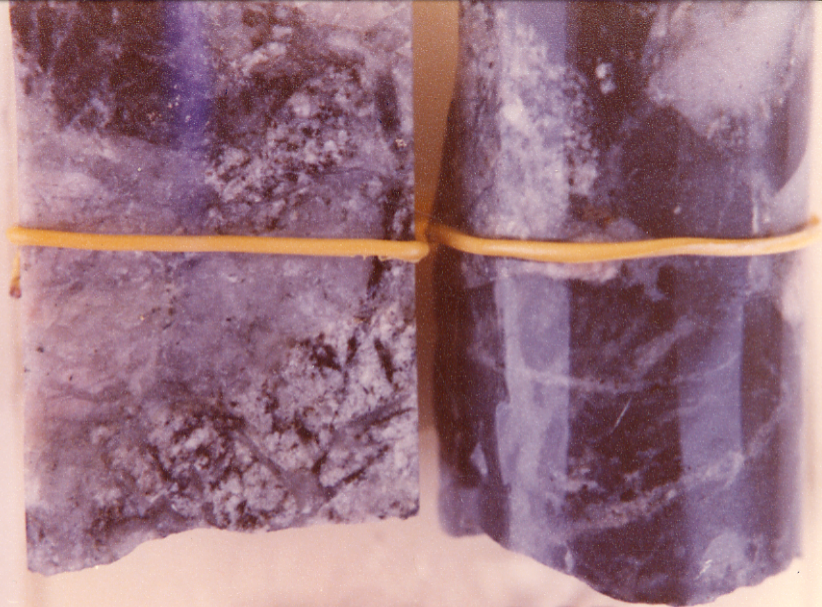
BRECCIA PIPE
