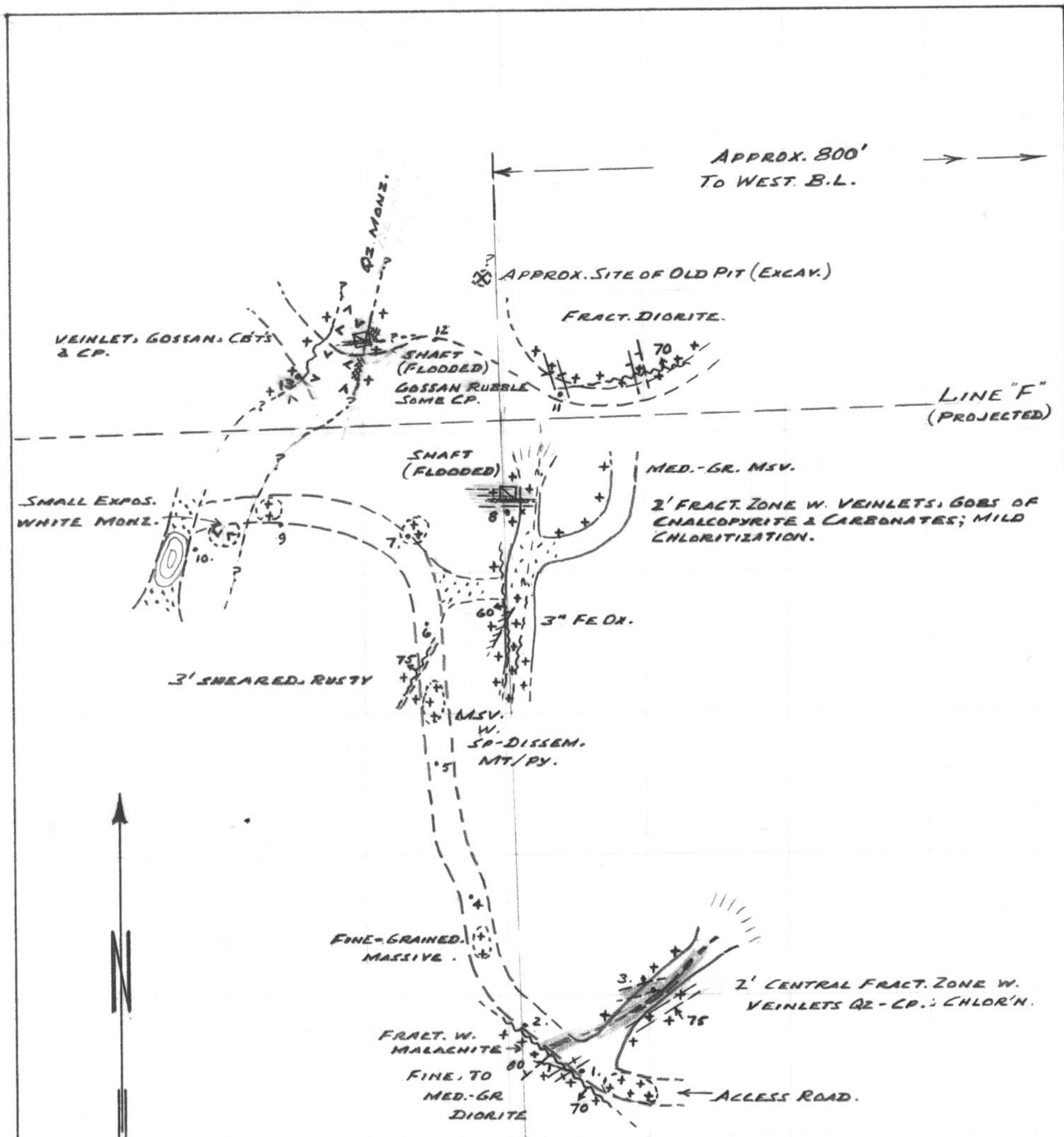
FIG. 4 A-1 WEST ZONE EXPLORATION. MAMIT LAKE MINING LTD. (N.P.L.) SCALE: 1" = 100' MAY, 1968
