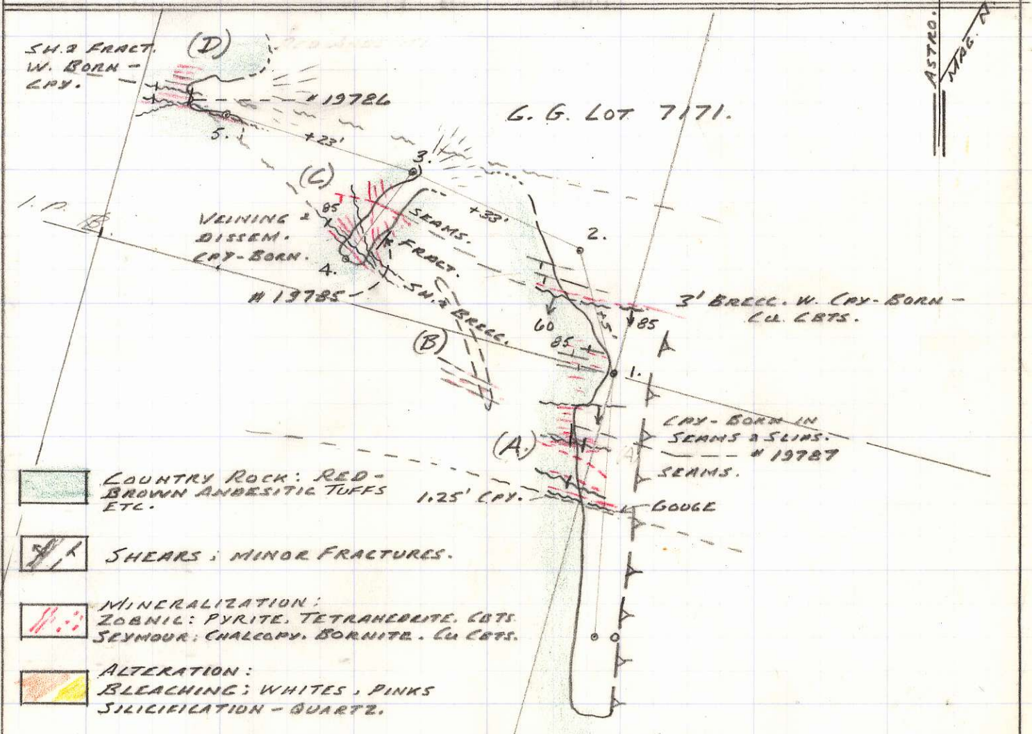
PLAN -- FIG. 2
