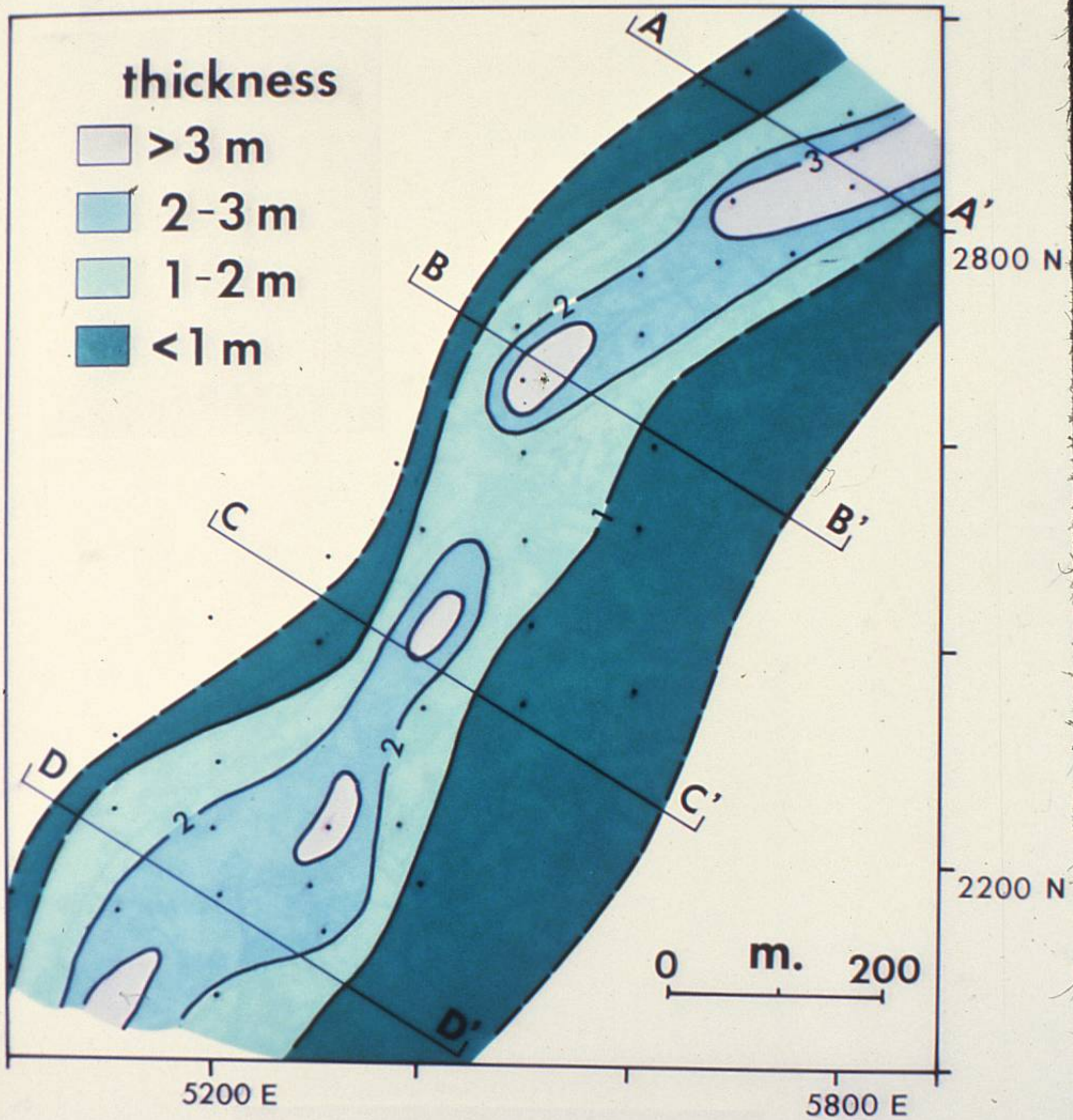
ISOPACH MAP
