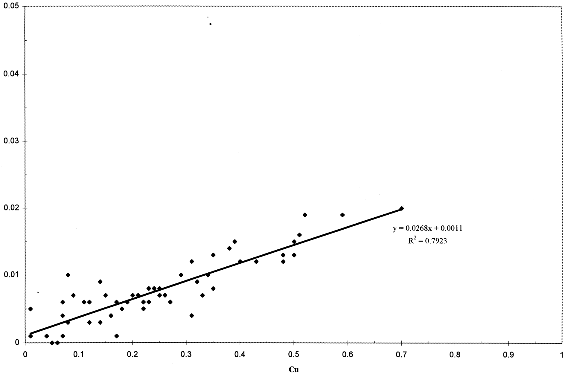
EC 98: Au vs. Cu Scatter
