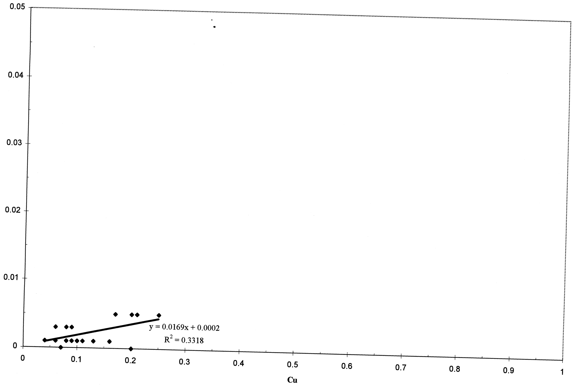
EC 77A: Au vs. Cu Scatter
