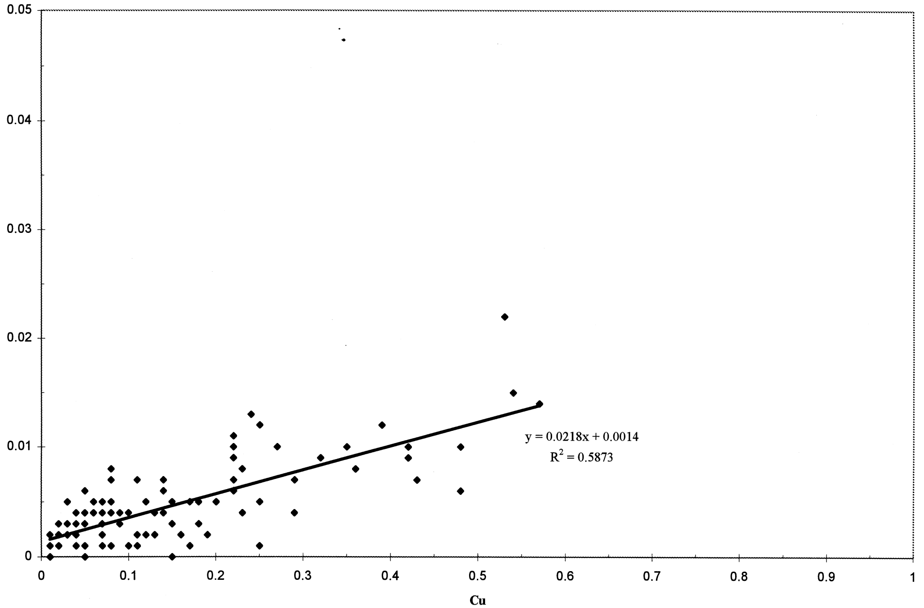
EC 187: Au vs. Cu Scatter
