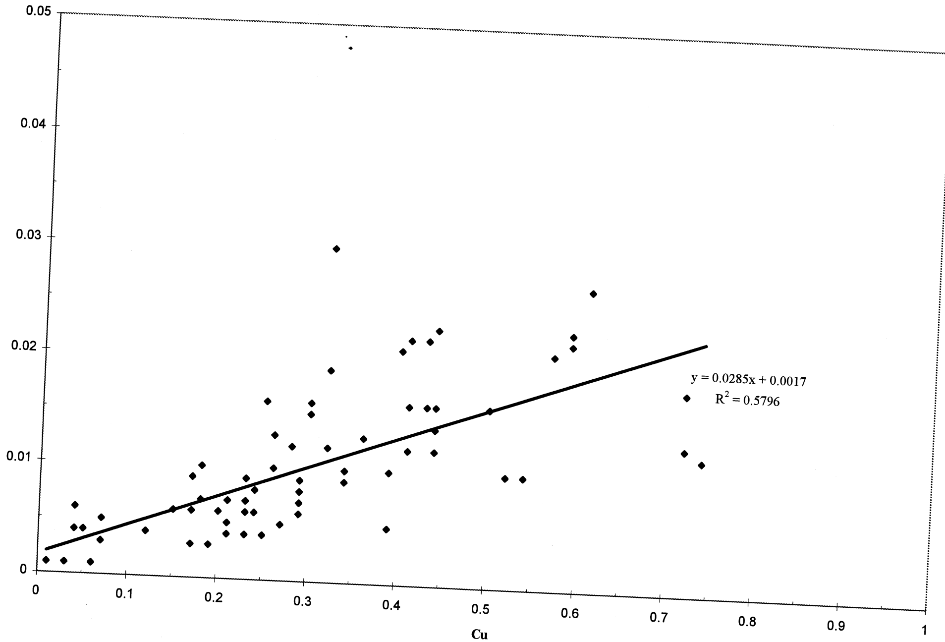
EC 100: Au vs. Cu Scatter
