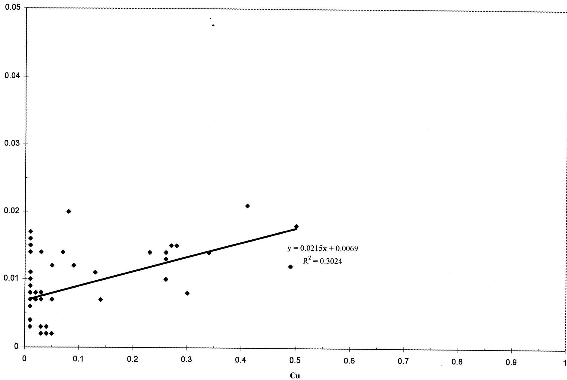
EC 86: Au vs. Cu Scatter
