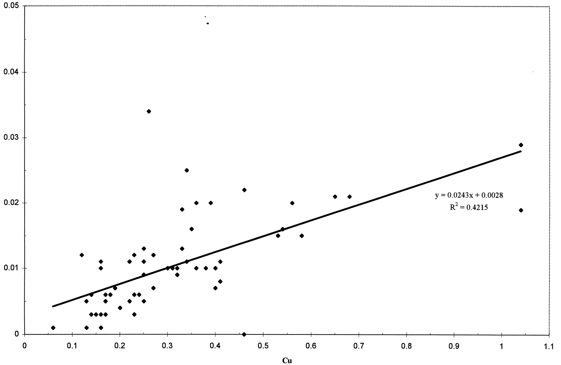
EC 105: Au vs. Cu Scatter
