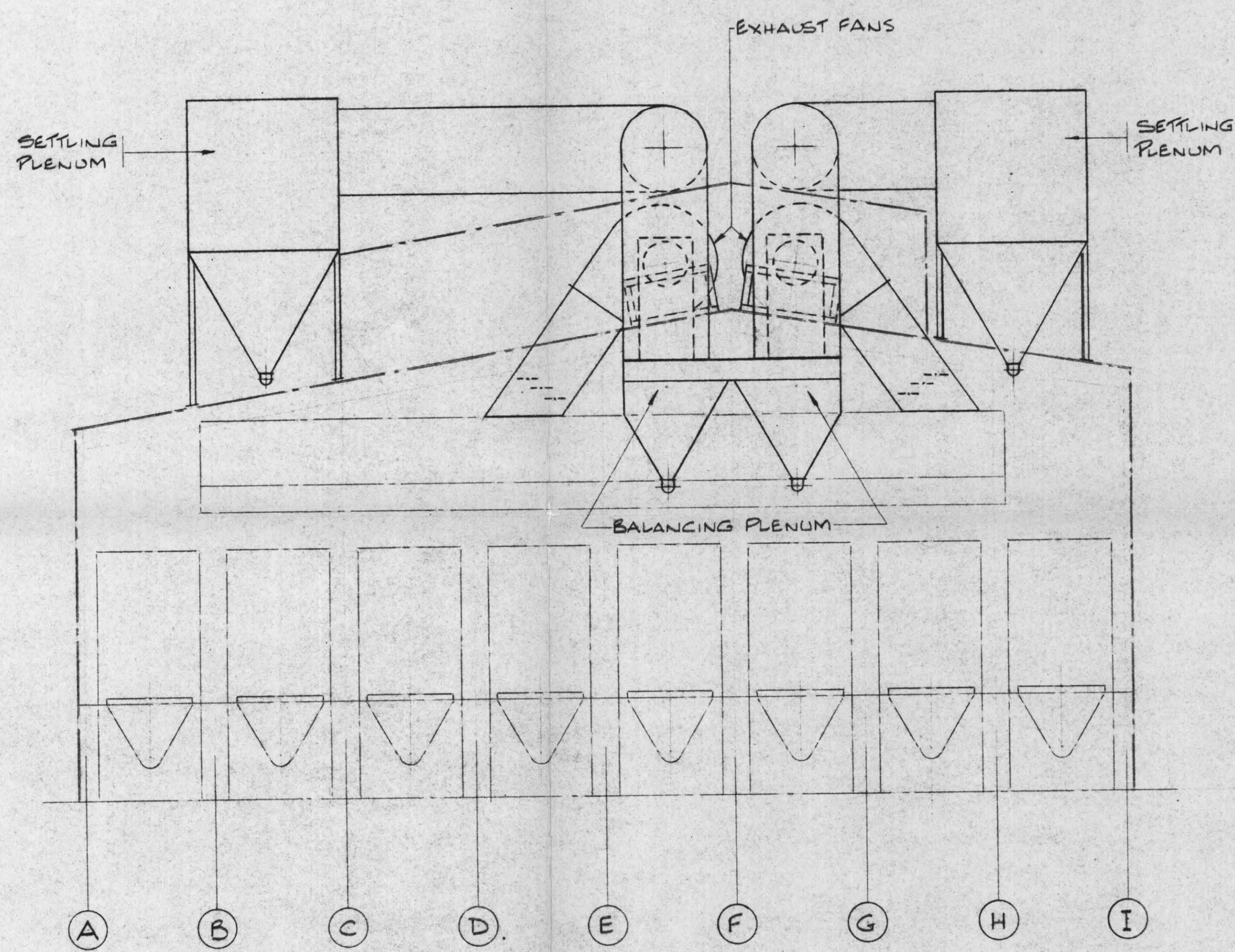
SECTION A-A
