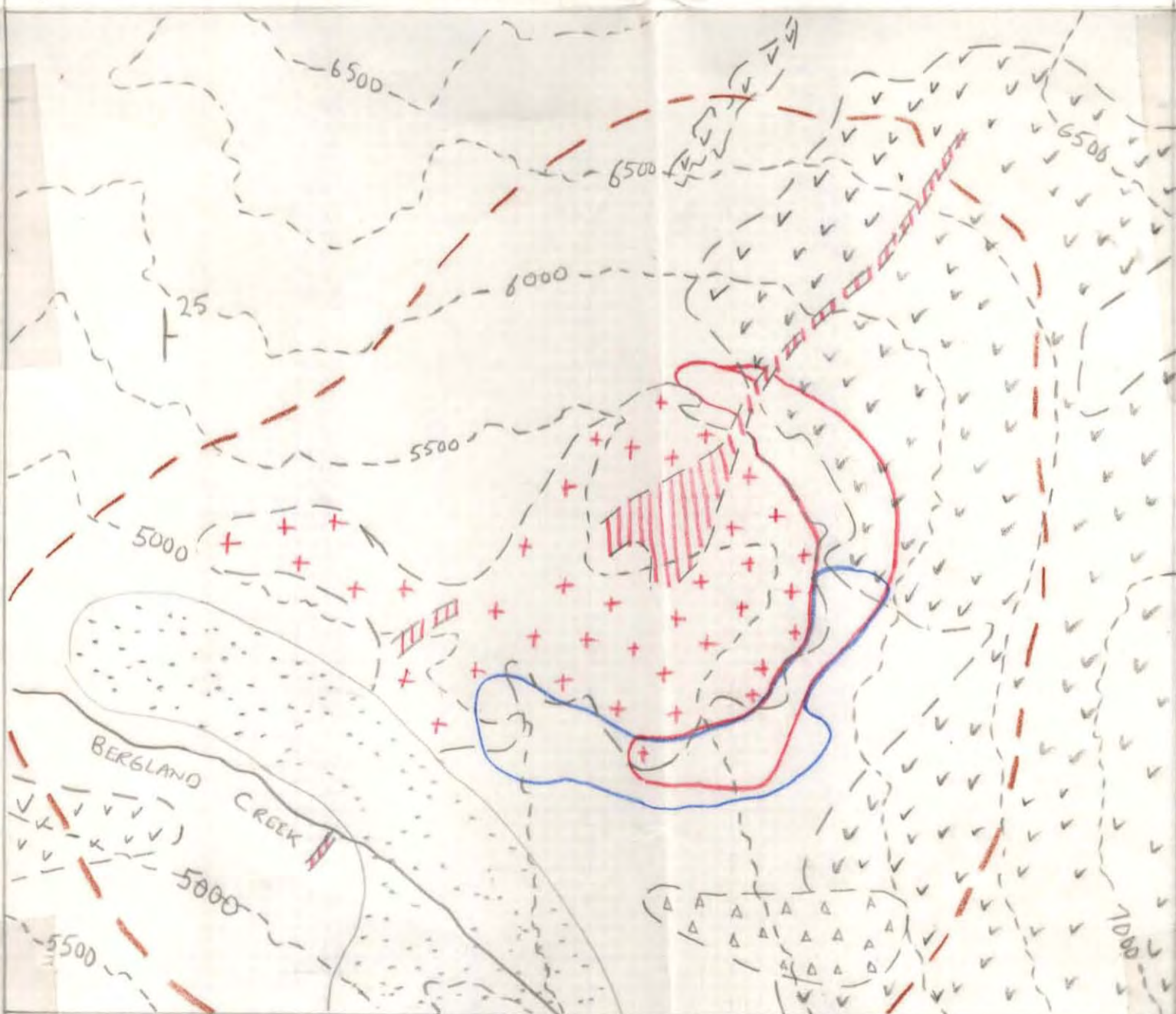
FIG. 11 GEOLOGY OF BERG PROSPECT
